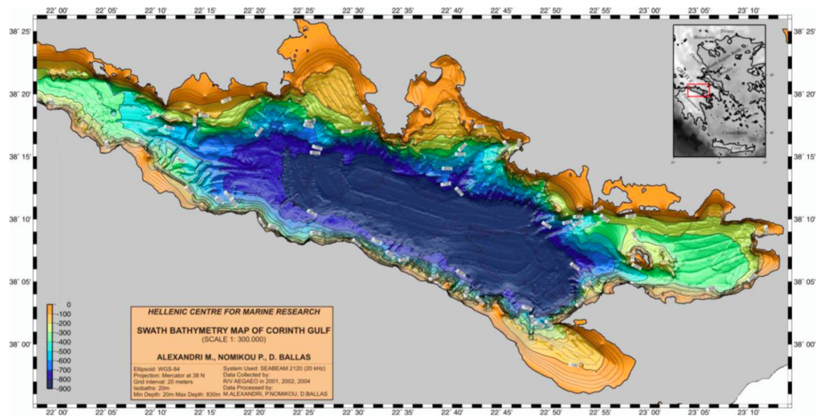
FIGURE 2.6 – Carte bathymétrique du rift de Corinthe. D'après Nomikou et al. [2011].
