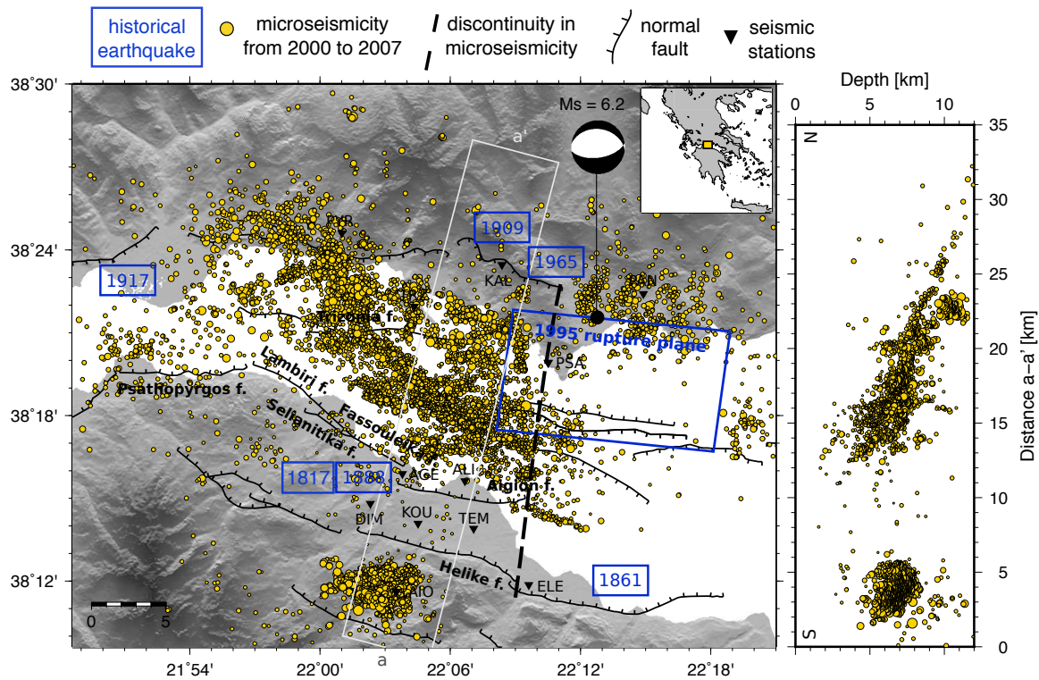
FIGURE 2.8 – Carte des derniers séismes historiques et de la microsismicité de la partie occidentale du rift de Corinthe entre 2000 et 2007. La microsismicité (jaune) a été enregistrée par le réseau CRL, Corinth Rift Laboratory (triangles noirs) et relocalisée par Lambotte et al. [2014] . Le mécanisme au foyer de composante normale est associé au séisme de 1995 de magnitude M_S = 6.2 Bernard et al. [1997] dont le plan en surface est délimité en bleu. Les séismes historiques [ Bernard et al., 1997 ; Papazachos et al., 1997 ] sont indiqués par leur date encadrée en bleu. Les failles sont les principales structures présentées dans Moretti et al. [2003] , Palyvos et al. [2005] et Ford et al. [2016] . La ligne en pointillé noir marque la discontinuité de sismicité entre la partie est et ouest du rift.
